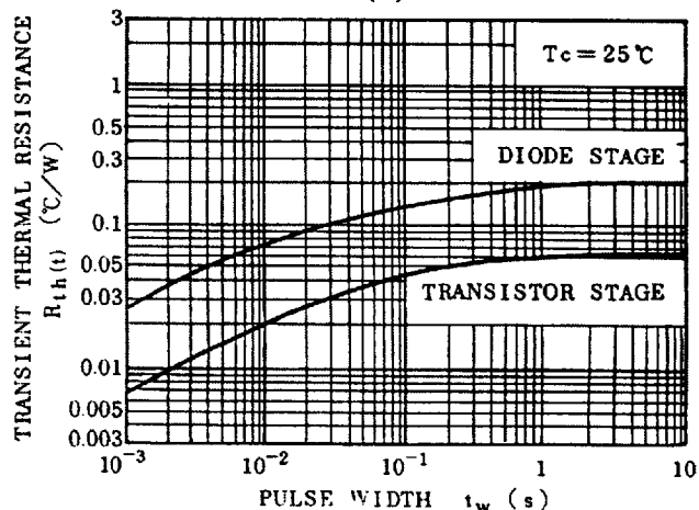
R_{th}(t) - t_w
