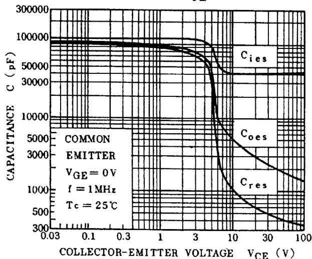
C - V_{CE}
